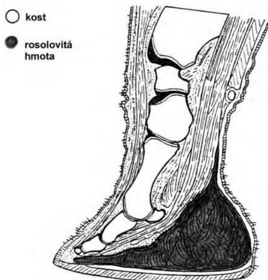
Obr. 107. Noha slona.
