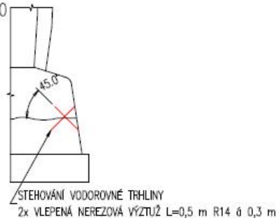
SCHÉMA STEHOVÁNÍ ZÁKLADOVÉHO BLOKU ŘEZ, M 1:50
