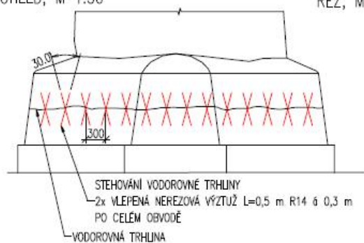
SCHÉMA STEHOVÁNÍ ZÁKLADOVÉHO BLOKU POHLED, M 1:50
